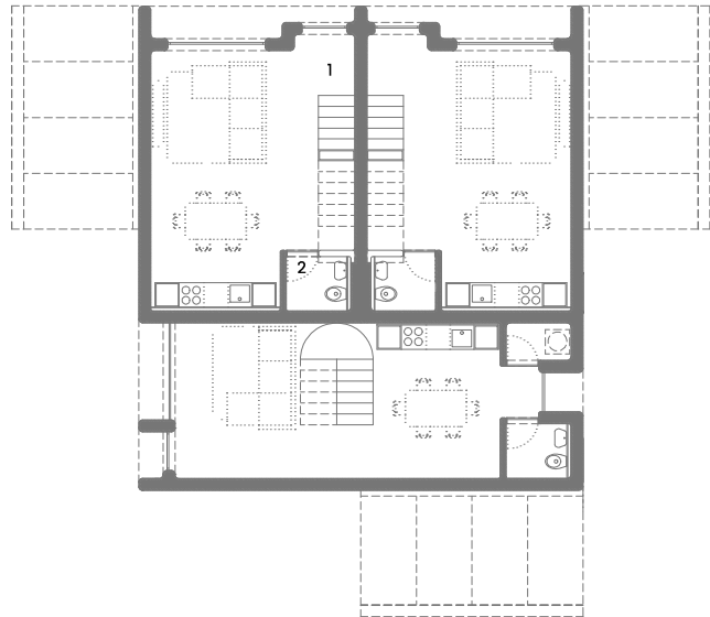
PLANTA DO PISO 1 esc: 1/200
