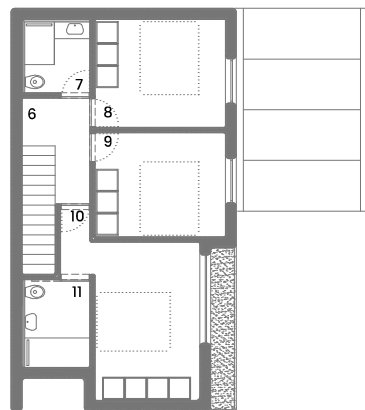
PLANTA DO PISO 2 esc: 1/200
